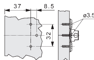
穴加工図
