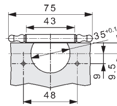
扉加工図 ネジ止め
