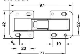
取付寸法図
