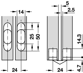
穴加工図
