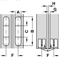
穴加工図
