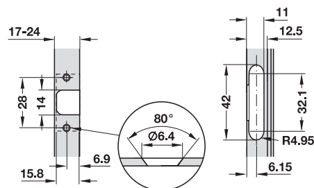
穴加工図
