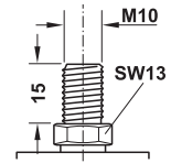
ネジ込みボルト、 スチール、 亜鉛メッキ
