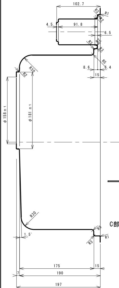
B-B断面図 1/3
