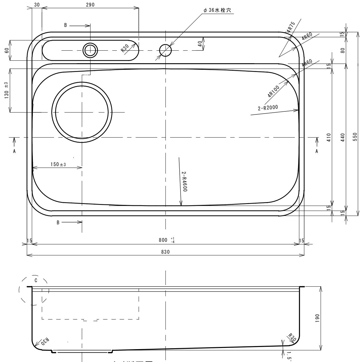
A-A断面図
