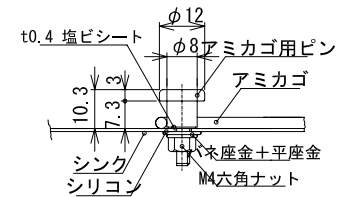
アミカゴ用ピン取付詳細 S = 1 / 2
