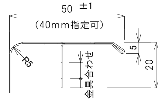
B-B'断面 S=1/1
