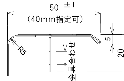
A-A'断面 S=1/1
