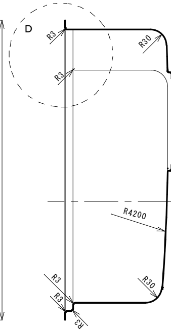
B-B断面図
