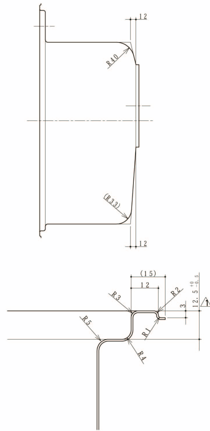
A 部詳細
