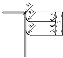
C部詳細 1/1
