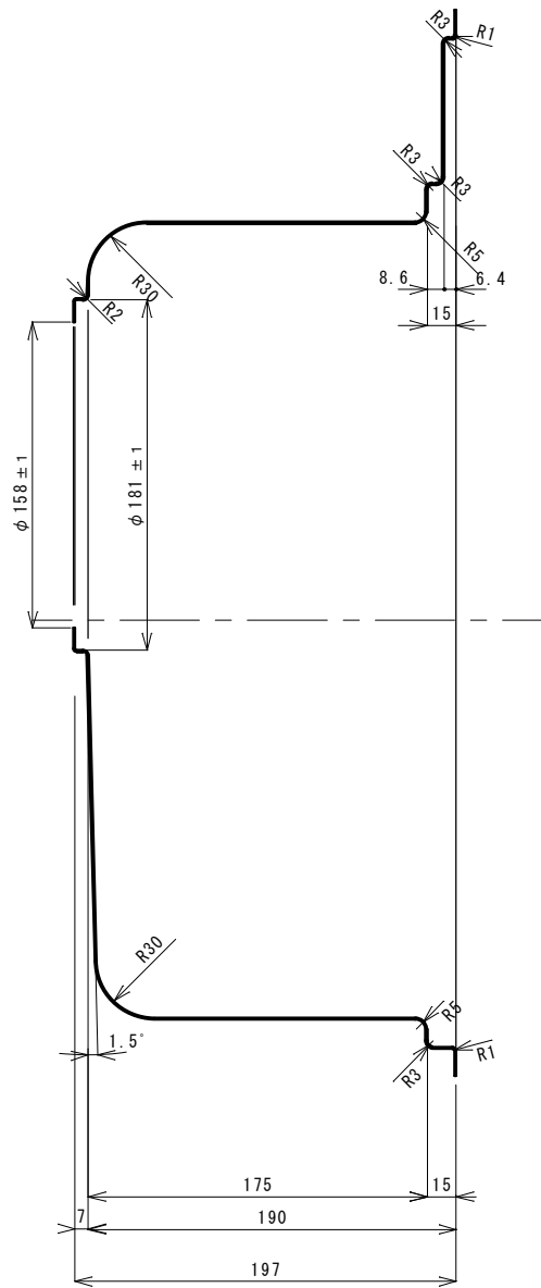
B-B断面図 1/3
