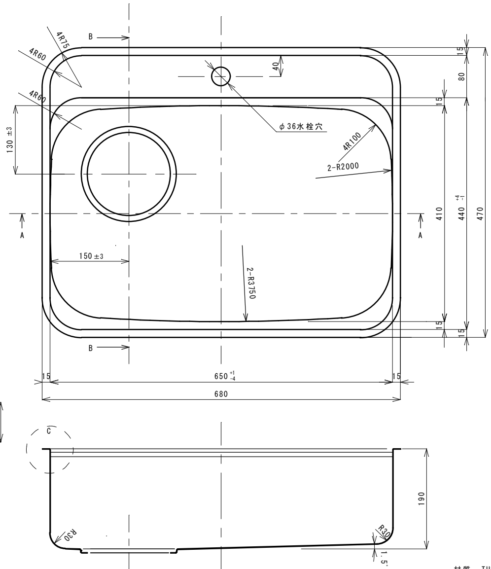
A-A断面図
