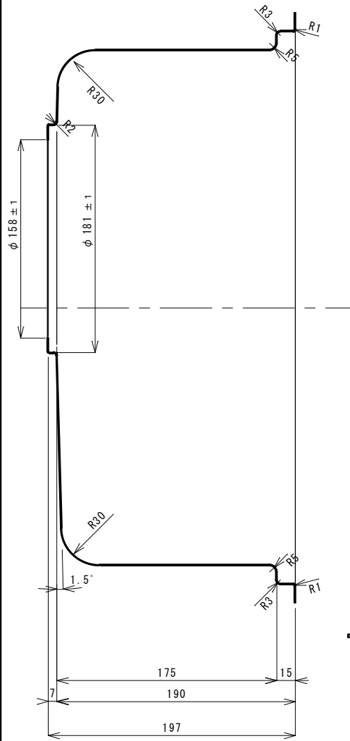
B-B断面図 1/3
