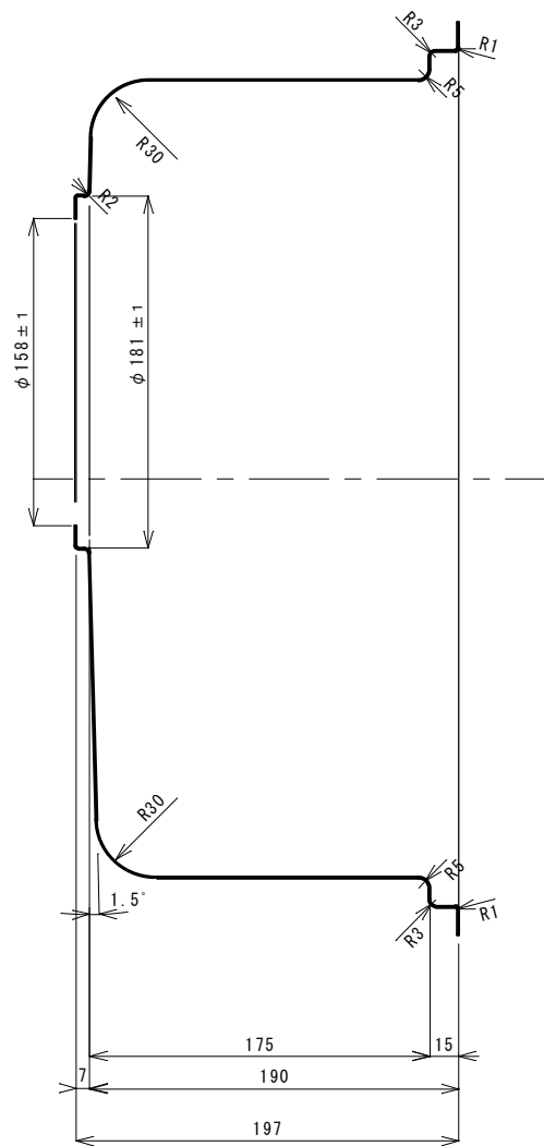
B-B断面図 1/3
