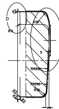
B-B 断面图
