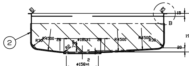
A-A 断面图
