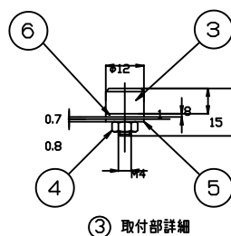
③ 取付部詳細
