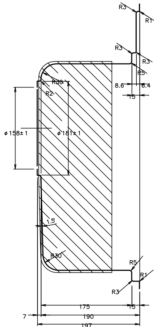
B-B 断面図(1/3)
