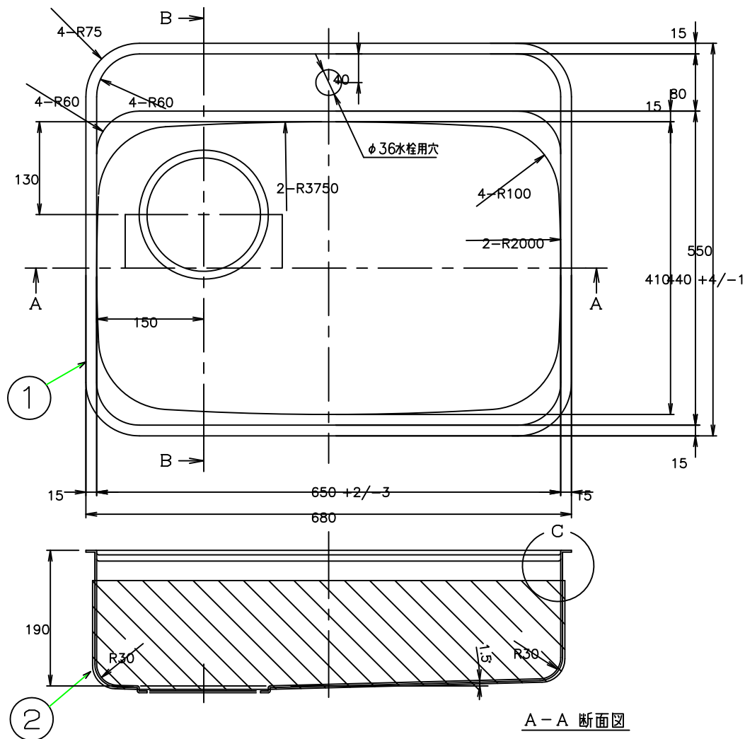
C 部詳細(1/1)
